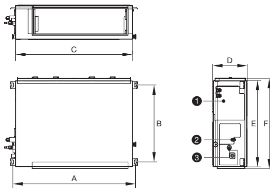
■ GUD71PH1/A-S - GUD160PH1/A-S
